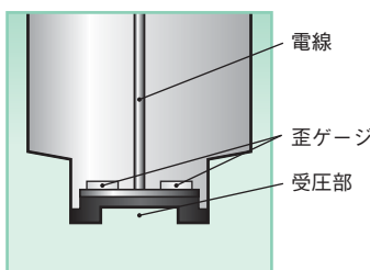
内部構造図
