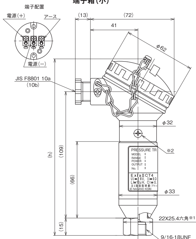
端子箱 (小)
