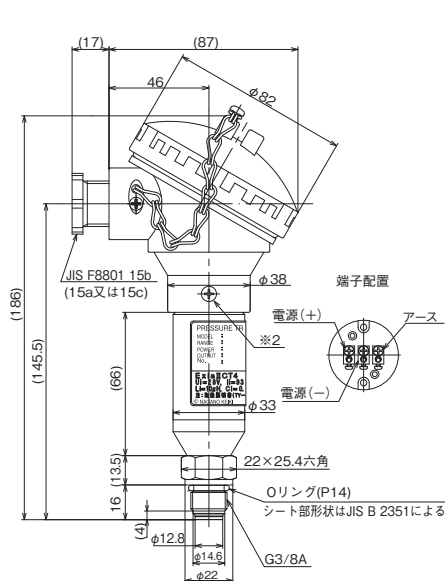
KJ16-9V4(端子箱式-大)
