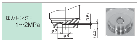
先端形状外形寸法図
